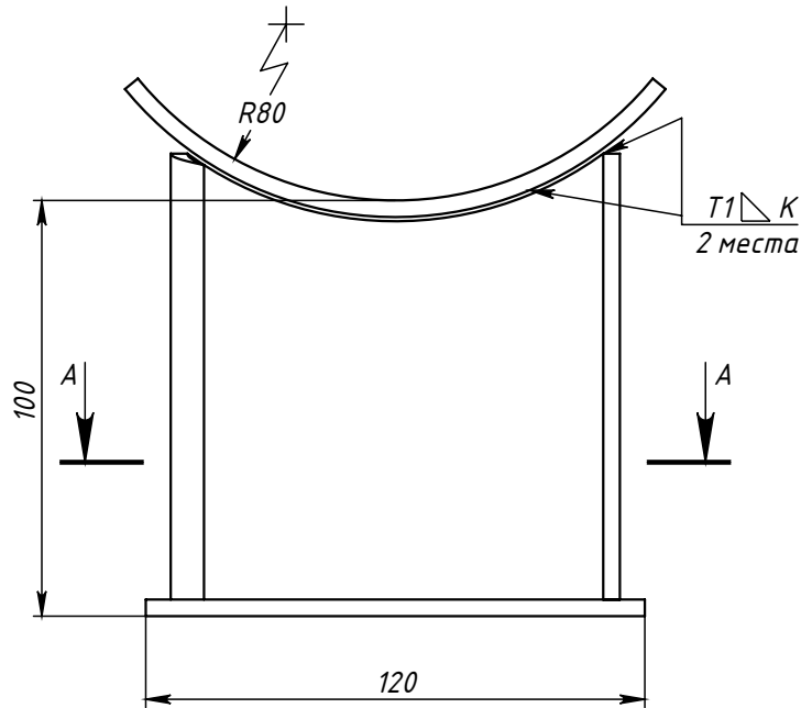
Поз.3 (Ложемент)
